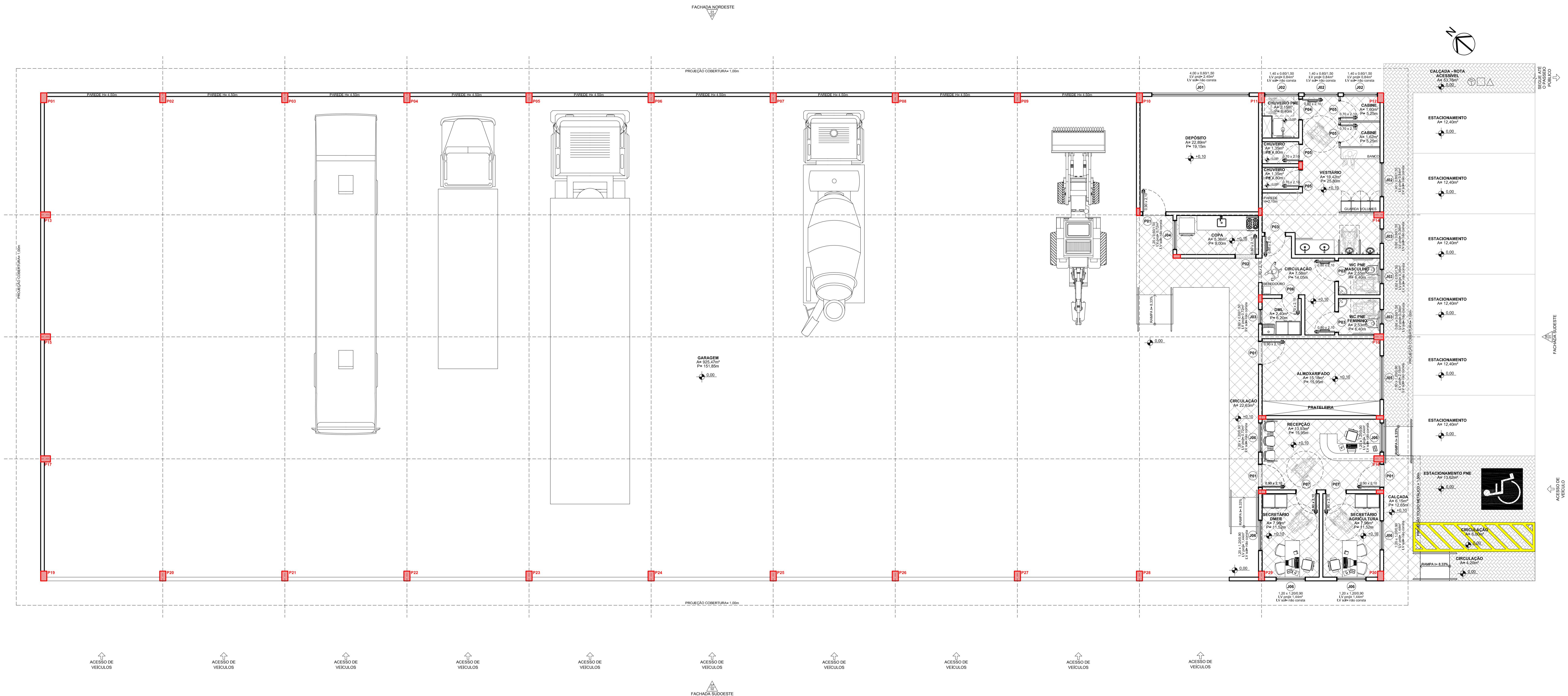
01 PLANTA BAIXA HUMANIZADA PAVIMENTO TÉRREO ESCALA: 1/75
