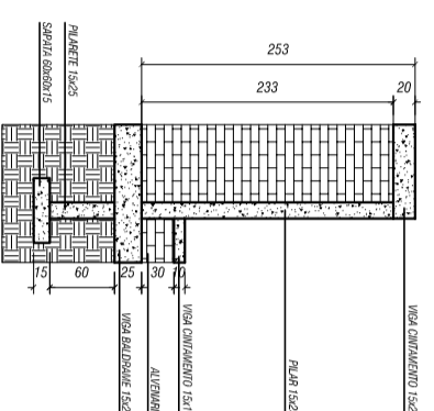
Detalhamento Estrutura Escala: 1:75
